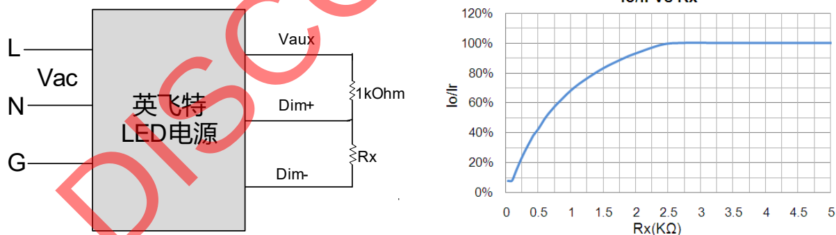
示意图 2: 电阻曲线
